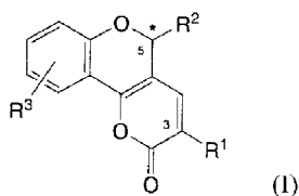
pyrano[3,2-c]chromén-2(5H)-ón
