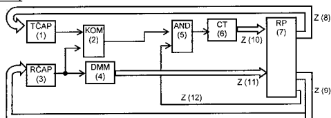
Obr. 1. Bloková schéma testera číslicovo-analógových prevodníkov
